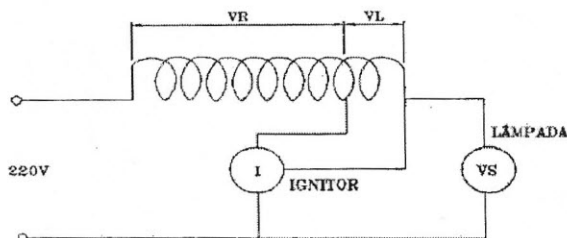
DETALHE 2
