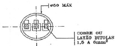
VISTA INFERIOR
